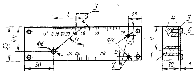
1 — отверстие для определения угла ввода луча, ширины основного лепестка диаграммы направленности, условной и предельной чувствительности; 2 — отверстия для проверки мертвой зоны; 3 — преобразователь; 4 — блок из контролируемого металла; 5 — шкала; 6 — винт
