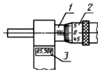
Цифровое устройство микрометров типов МВМЦ, МВТЦ, МВПЦ
