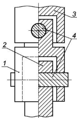
Рисунок К.5 - Схема шарнира Гука
