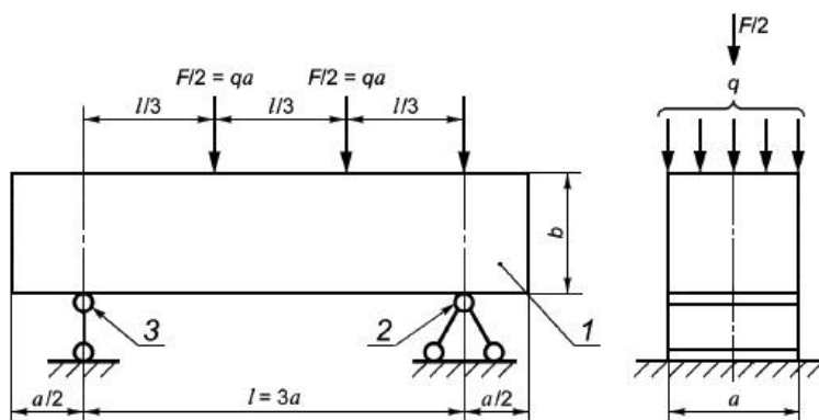
Рисунок 2 - Схема испытания на растяжение при изгибе
