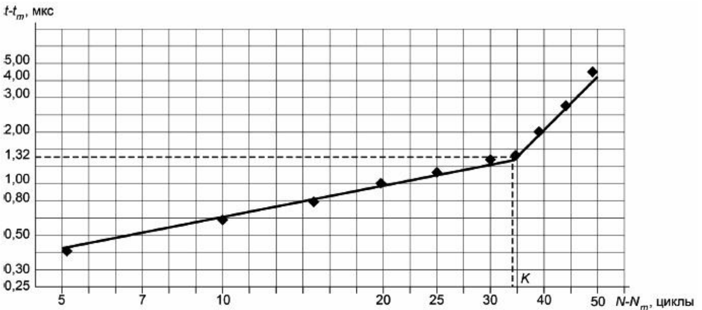
Рисунок Д.1 - График ультразвуковых измерений образца N 1
