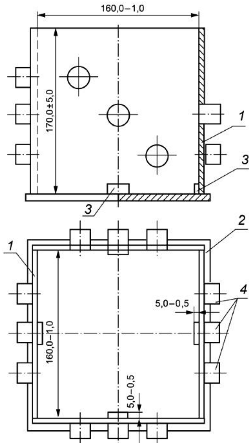
Рисунок В.1 - Схема испытательной ванны для образцов размерами 150x150x150 мм
