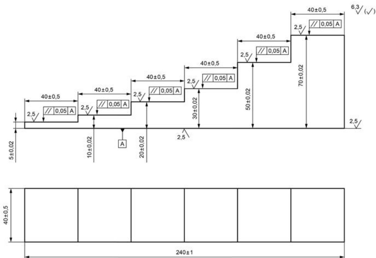
Рисунок 19 - Настрочный образец толщины НОТ-1
