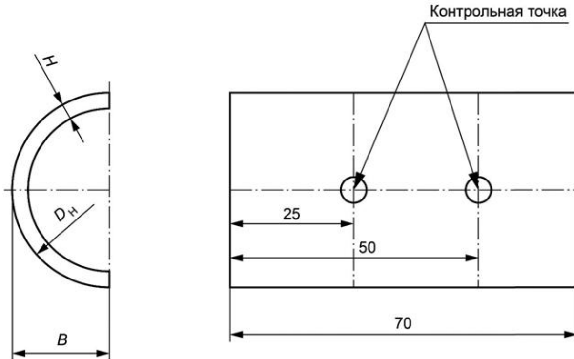
Рисунок 17 - Настроечный образец в виде участка трубы
