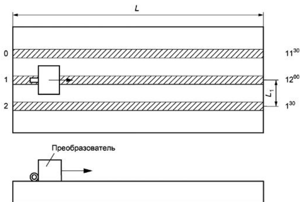
Рисунок 8 - УЗКТ непрерывным сканированием по полосам (линиям)
