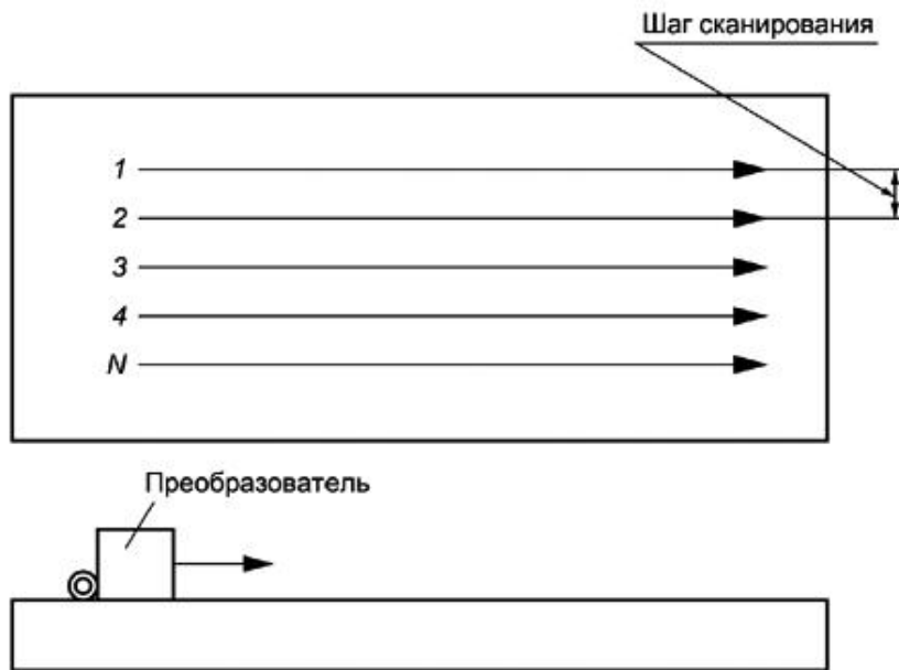
Рисунок 9 - УЗКТ непрерывным сканированием участка поверхности
