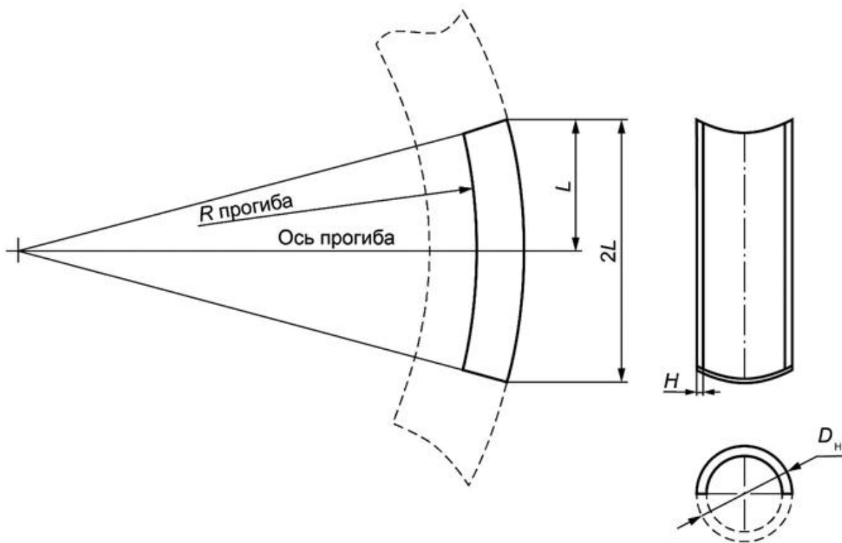
Рисунок 18 - Настроечный образец в виде участкагиба (колена) трубопровода
