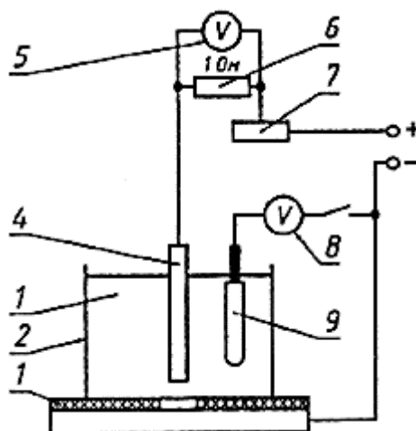
Рисунок В.3 - Схема проведения испытания образцов покрытий на пластинах (картах) для определения площади отслаивания с применением магниевого анода
