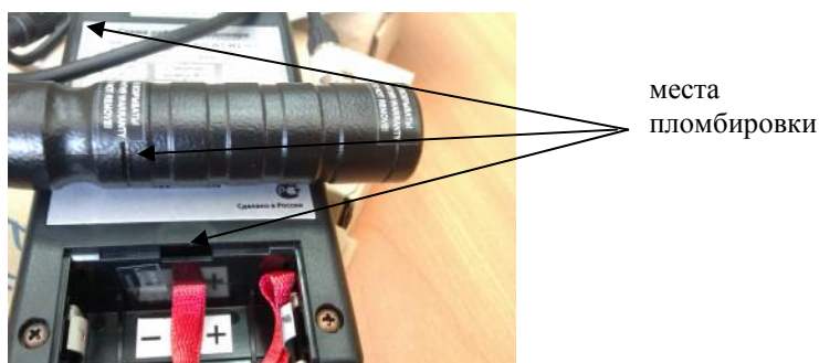
Рисунок 2 - Схема пломбировки твердомера.
