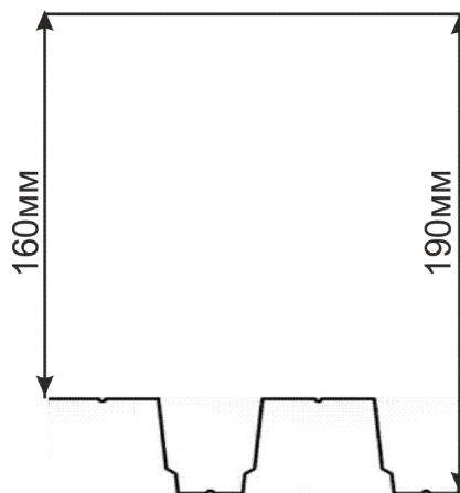
Эскиз железобетонного перекрытия с несъемной опалубкой
