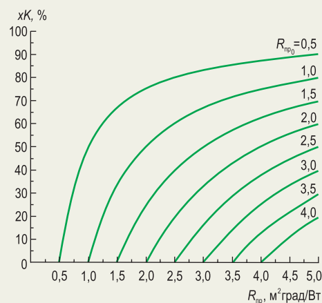
Рис. 2. Зависимость относительных теплопотерь xK от приведенного сопротивления теплопередаче R_{пр} для разных начальных значений сопротивления теплопередаче ( K – коэффициент нормировки, равный 0,32; 0,29; 0,24; 0,09 и 0,08 для стен, окон, кровли, воздухообмена и фундамента соответственно)
