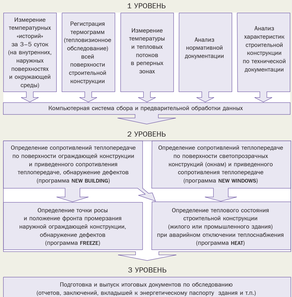
Рис. 4. Структурная схема комплексного тепловизионного контроля зданий и строительных конструкций (в летний и зимний периоды)
