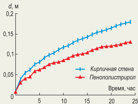
Рис. 3. Движение границы промерзания по толщине d однородной стены из кирпича и пенополистирола с учетом скачкообразного изменения теплоемкости на границе
