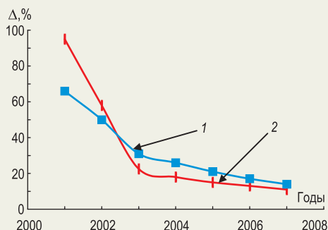
Рис. 1. Изменение доли \Delta объектов, не соответствующих нормам энергосбережения, после введения обследований тепловизионным методом с прогнозированием результатов: 1 – административные здания; 2 – жилые здания
