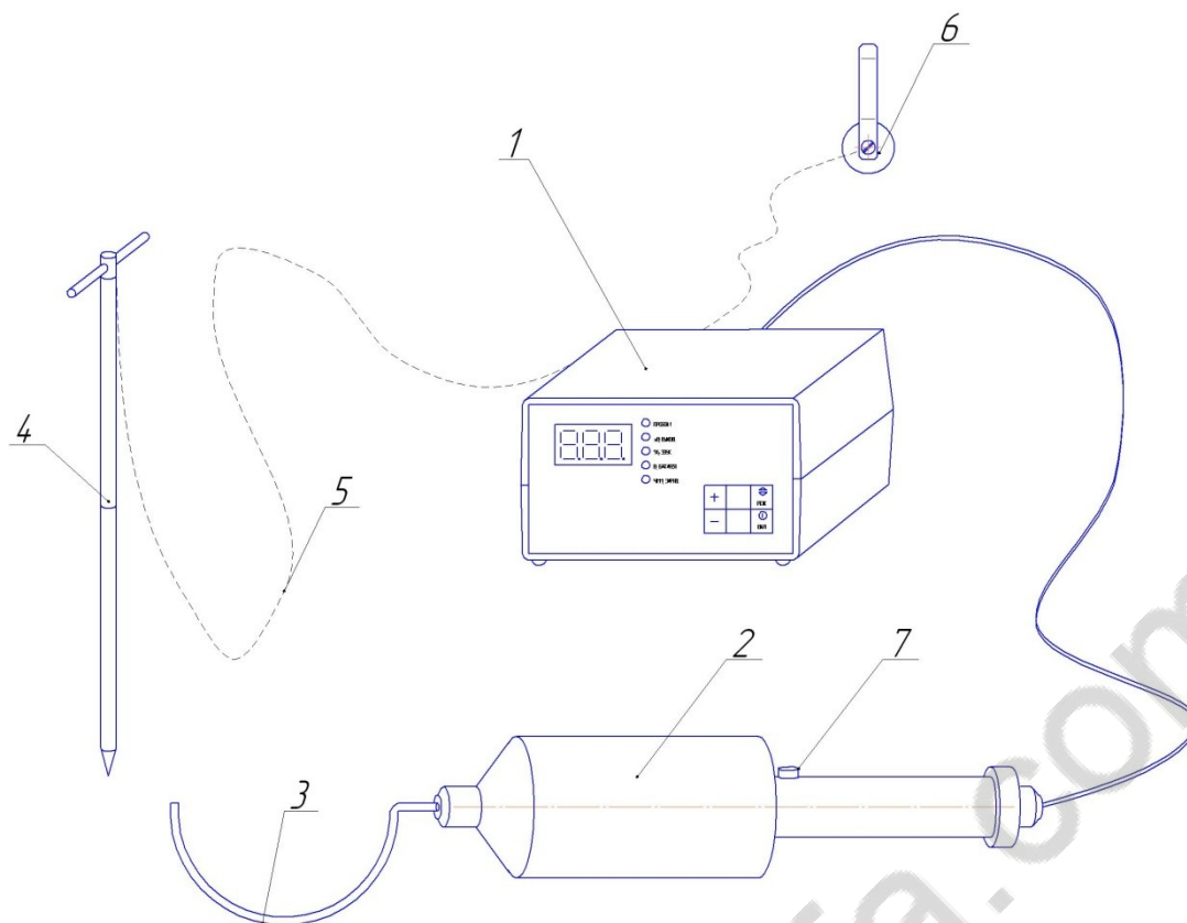
Рис.1. Комплект ДКИ-3К.
