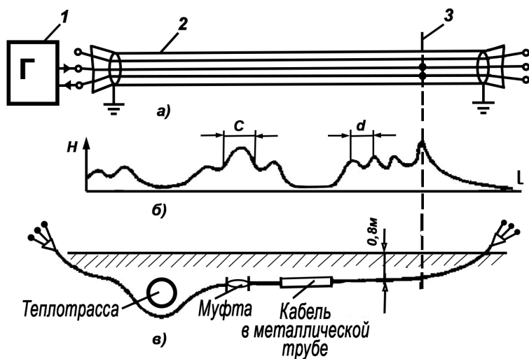
Рис.9.10 КЗ-междуфазное
